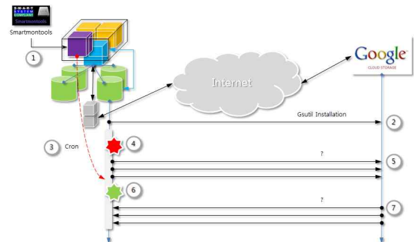
그림 10. Google Storage를 이용한 SD RAID 기반 장애복구 모듈의 시스템 환경.
