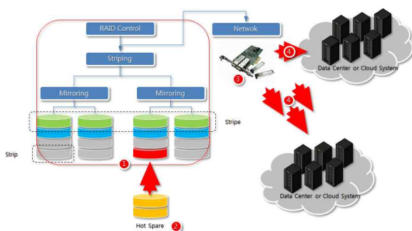
그림 3. Software Defined Storing 기술의 개념도
