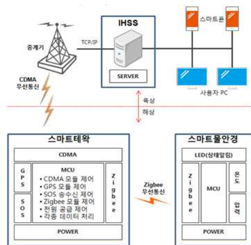
그림 1. Haenyeo Monitoring System 구성도
