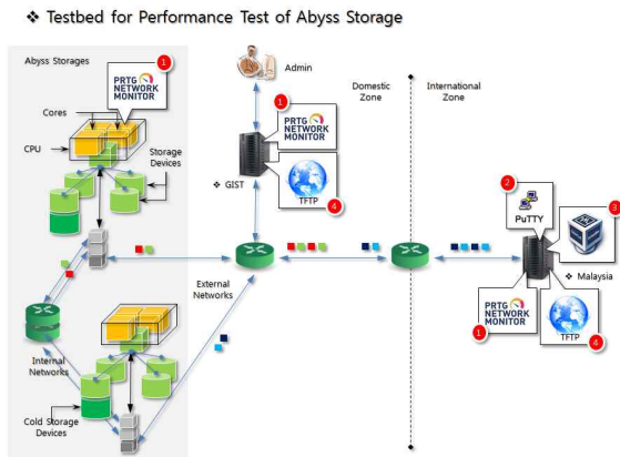
그림 15. 실환경 성능 테스트를 위한 테스트베드 구성도
