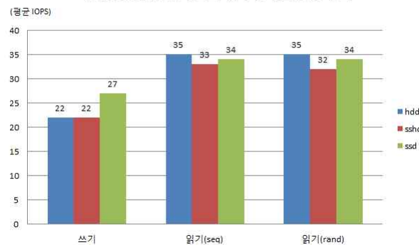
그림 10. 디스크 매체에 따른 IOPS 성능 비교
