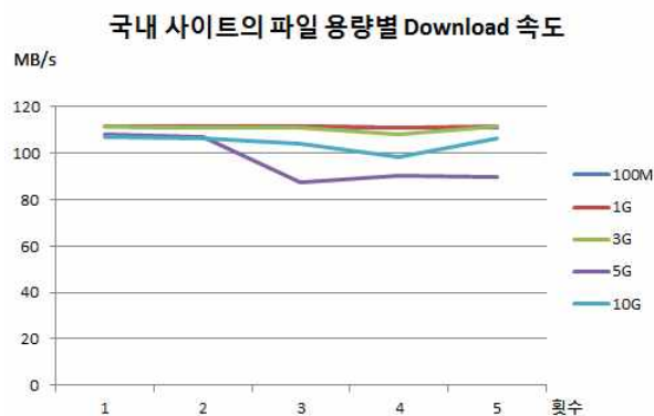
그림 16. GIST와 Abyss Storage의 Download 속도 측정
