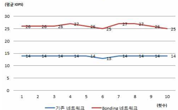
그림 12. 네트워크 본딩에 의한 Write의 IOPS 비교
