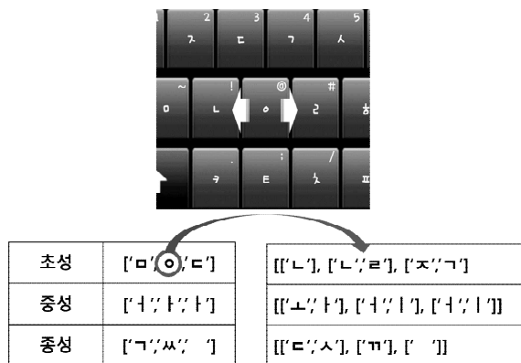
그림 2 자소 분리와 후보 목록 생성
