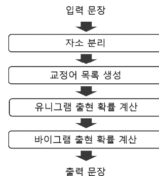
그림 1 오타 교정 과정
