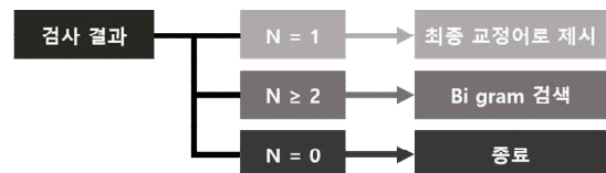
그림 4 유니그램 출현 빈도 검사 결과에 따른 선택
