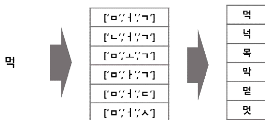
그림 3 교정 후보 초, 중, 종성의 결합
