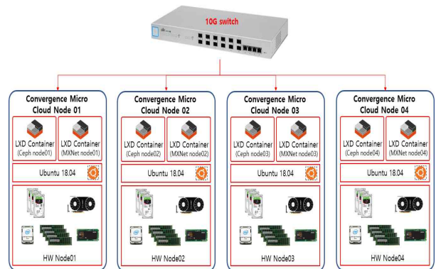
그림 7. 스토리지와 인공지능이 융합된 마이크로 클라우드 인프라의 개념도
