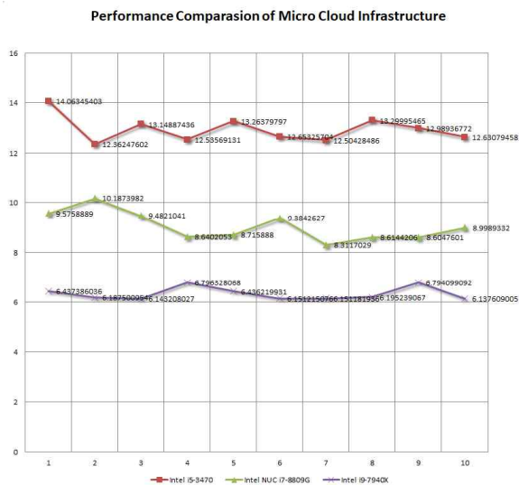
그림 9. 마이크로 클라우드 인프라의 성능 테스트 결과
