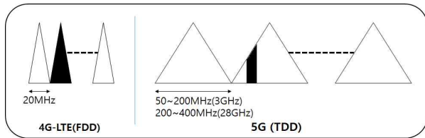
그림 2. FDD방식과 TDD방식의 비교[10]
