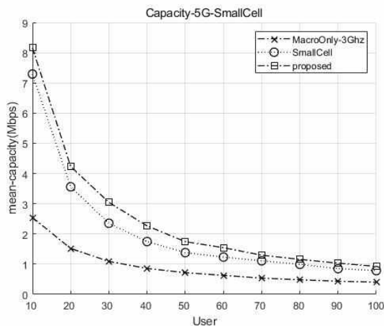
그림 7. 유저수증가에 따른 성능 비교
