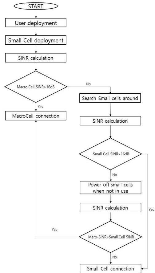
그림 7. 시나리오2 : 5G매크로 시스템 간섭제어 알고리즘
