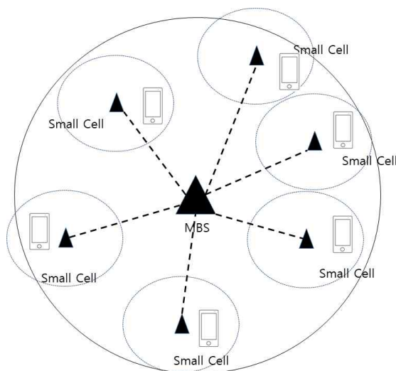
그림 2. 스몰셀 망 구조
