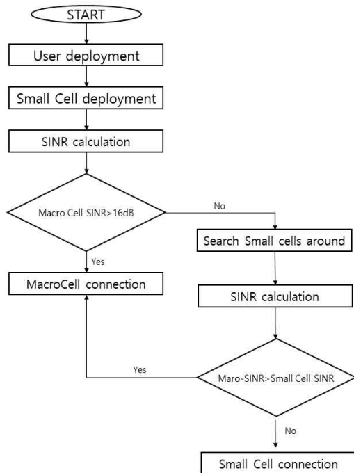
그림 6. 시나리오1 : 5G매크로 시스템 스몰셀 적용 알고리즘
