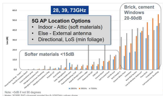
그림 1. 밀리미터파의 매질에 따른 신호감쇄[4]
