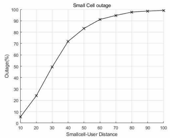
그림 5. 스몰셀과 유저간 거리에 따른 Outage
