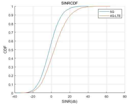
그림 4. 5G, 4G SINR CDF
