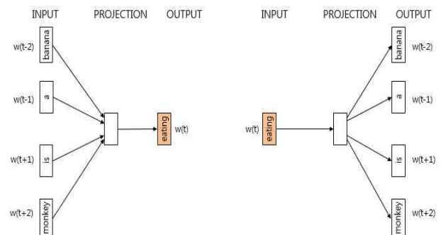
그림 2. CBOW 모델과 Skip-gram 모델
