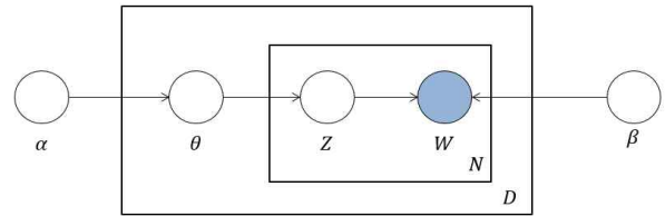
그림 1. LDA Model
